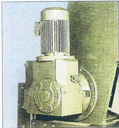
Groupe motoreducteur Usocom. Reduction gear assembly.
